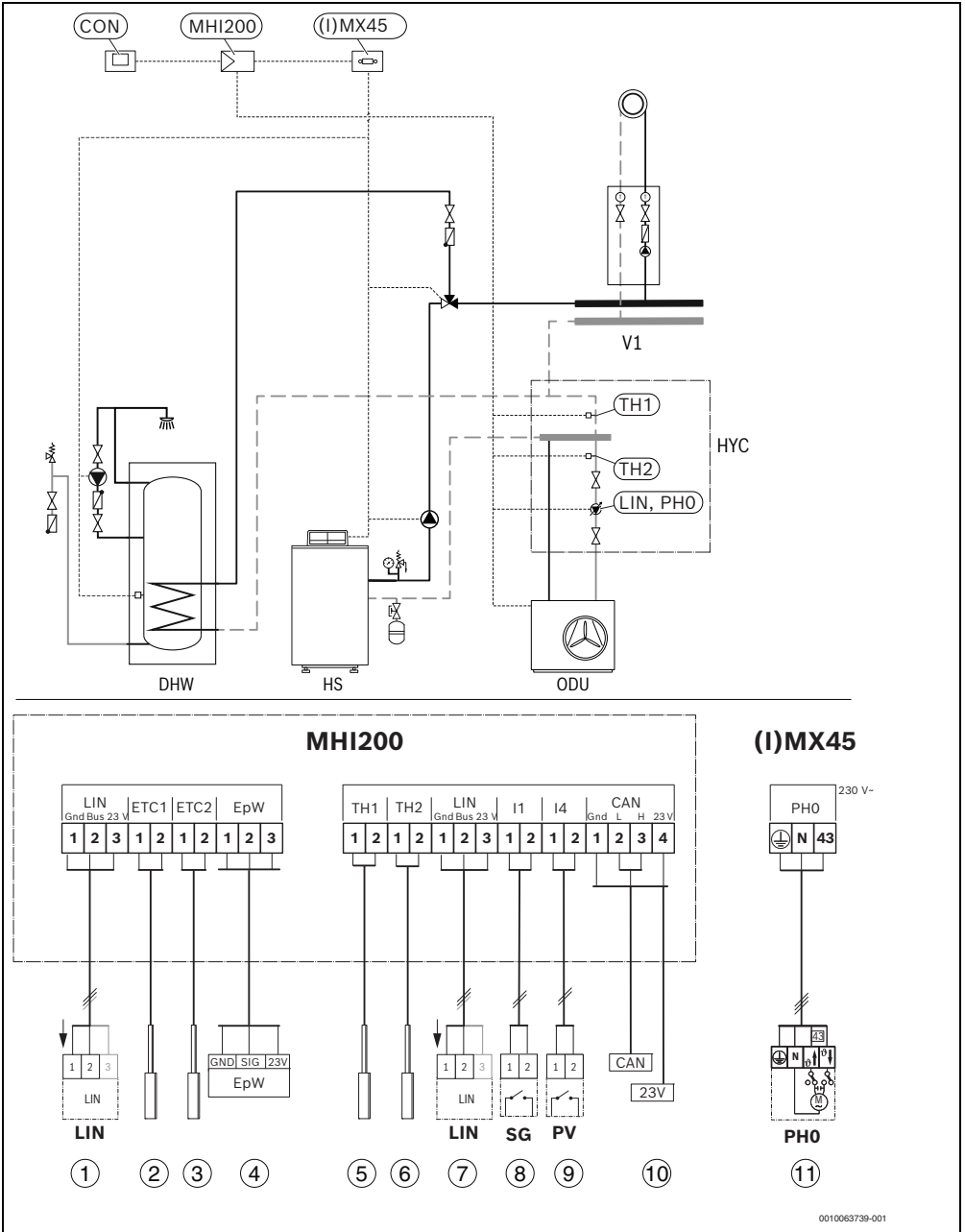
Afb. 26 Voorbeeld hydraulisch systeem: Hybride systeem met vloerstaande cv-ketel, warm water via driewegklep en systeem-pomp, 1 ongemengd cv-circuit
