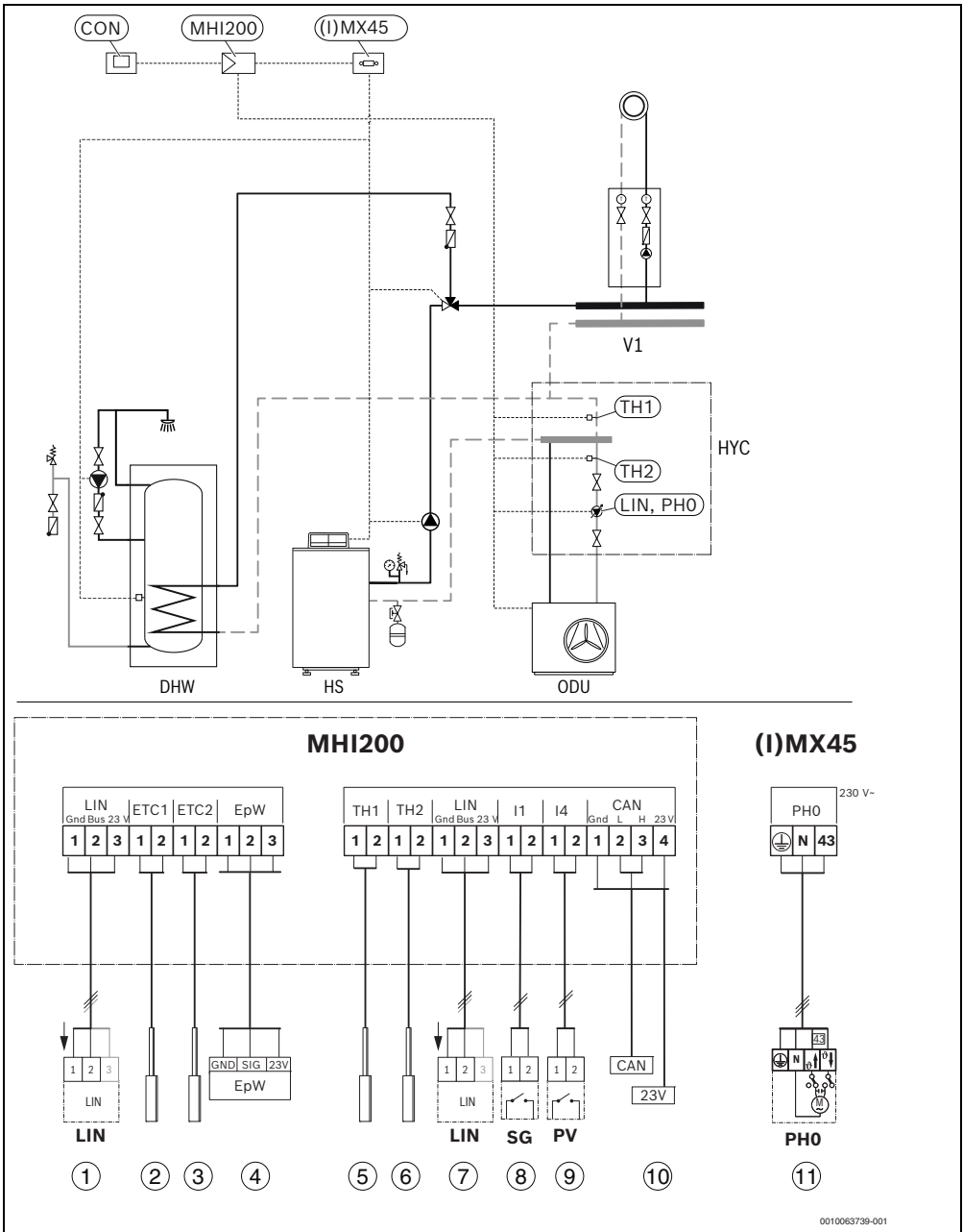
Bild 5 Beispiel Hydraulik: Hybridsystem mit bodenstehendem Kessel, Warmwasser über Dreivegeventil und Systempumpe, 1 gemischer Heizkreis
