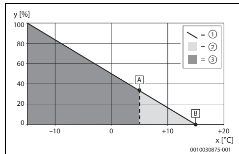
Fig. 16 Temperatura esterna alternativa
