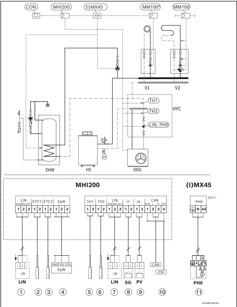
Fig. 11 Exemple de système hydraulique : système hybride avec générateur de chaleur au sol, eau chaude sanitaire sur la chaudière via pompe à charge et 1-4 circuits de chauffage mélangés
