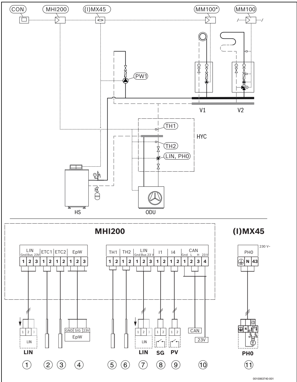
Fig. 20 Esempio di circuito idraulico: sistema ibrido con generatore di calore a basamento e bypass, nessuna produzione di acqua calda sanitaria e 1-4 circuiti di riscaldamento miscelati
