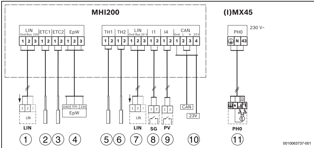
Afb. 24 Overzicht bezetting aansluitklemmen
