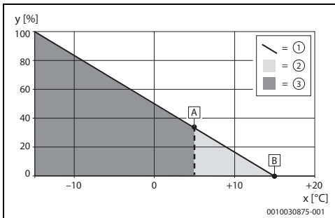
Bild 2 Außentemperatur alternativ
