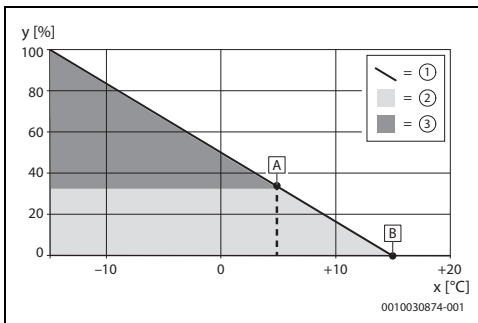
Fig. 8 Température extérieure parallèle
