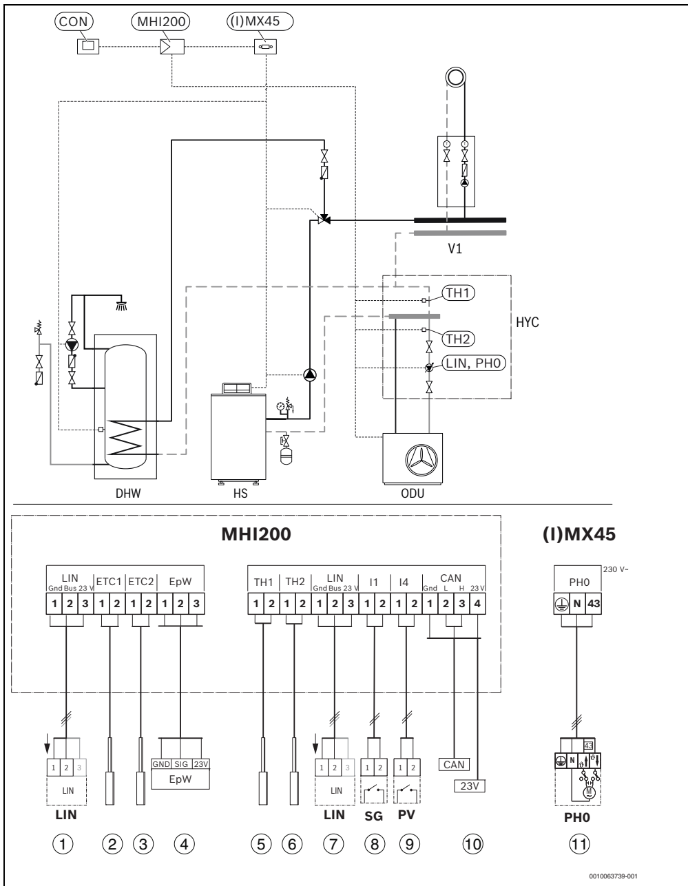
Fig. 19 Esempio di circuito idraulico: sistema ibrido con generatore di calore a basamento, produzione di acqua calda sanitaria mediante valvola a tre vie e circolatore di sistema, 1 circuito di riscaldamento miscelato
