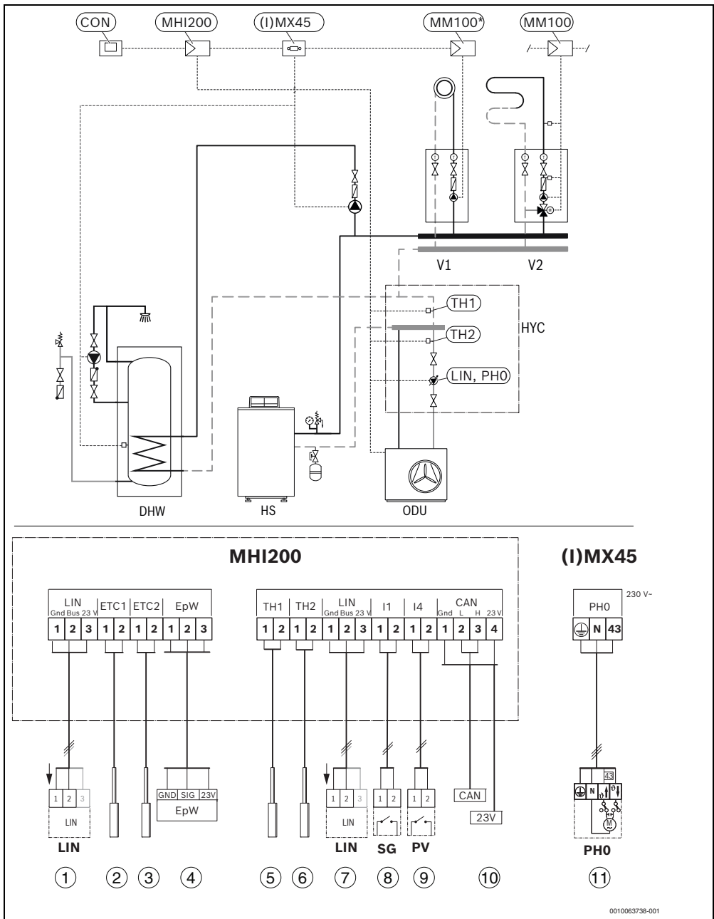
Fig. 18 Esempio di circuito idraulico: sistema ibrido con generatore di calore a basamento, produzione di acqua calda sanitaria con il generatore di calore mediante pompa di carico bollitore e 1-4 circuiti di riscaldamento miscelati
