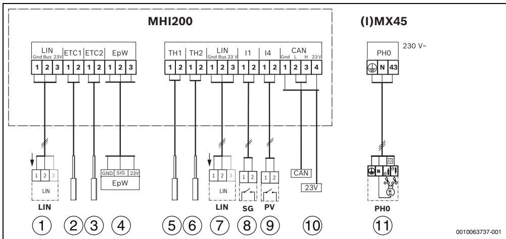
Fig. 10 Aperçu attribution bornes de raccordement
