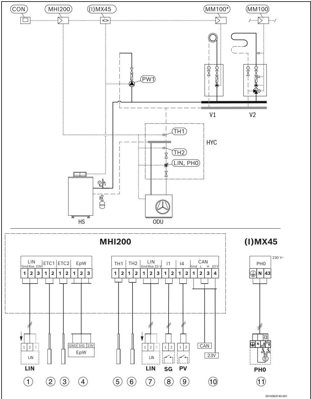
Afb. 27 Voorbeeld hydraulisch systeem: Hybride systeem met vloerstaande cv-ketel en bypass, geen warmwaterbereiding en 1-4 gemengde cv-circuits
