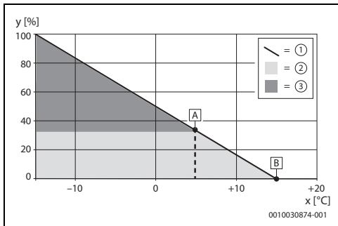
Fig. 15 Temperatura esterna parallela
