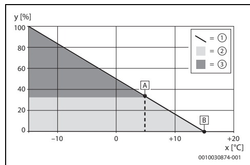
Afb. 22 Buitentemperatuur parallel
