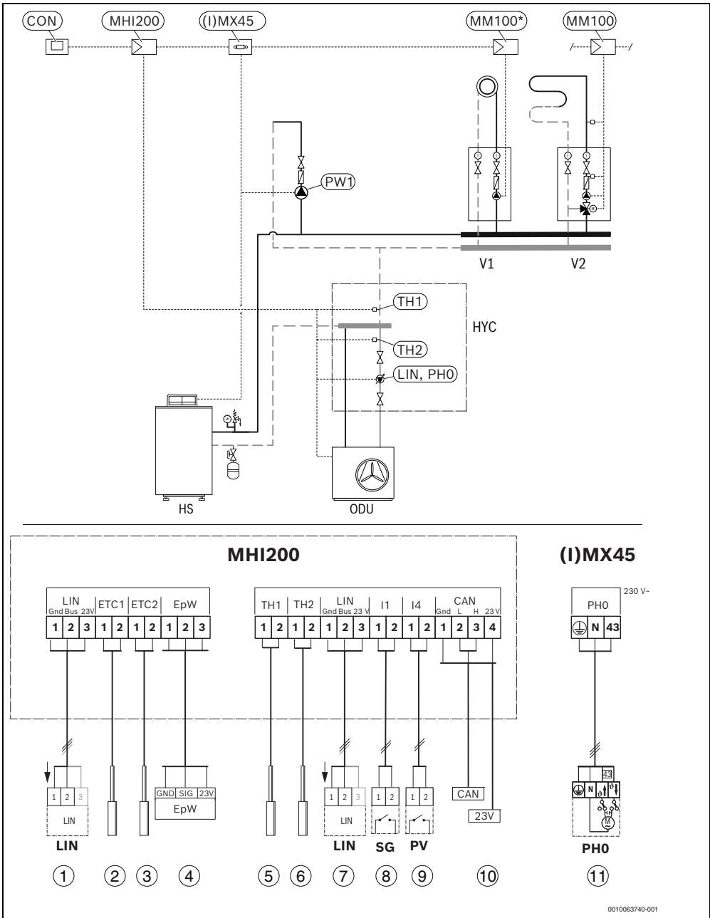
Fig. 13 Exemple de système hydraulique : système hybride avec chaudière au sol et by-pass, pas de production d'eau chaude sanitaire et 1-4 circuits de chauffage mélangés
