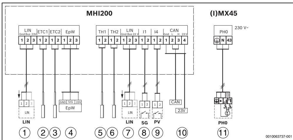
Fig. 17 Panoramica dei morsetti
