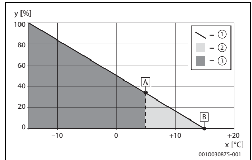
Afb. 23 Buitemtemperatuur alternatief
