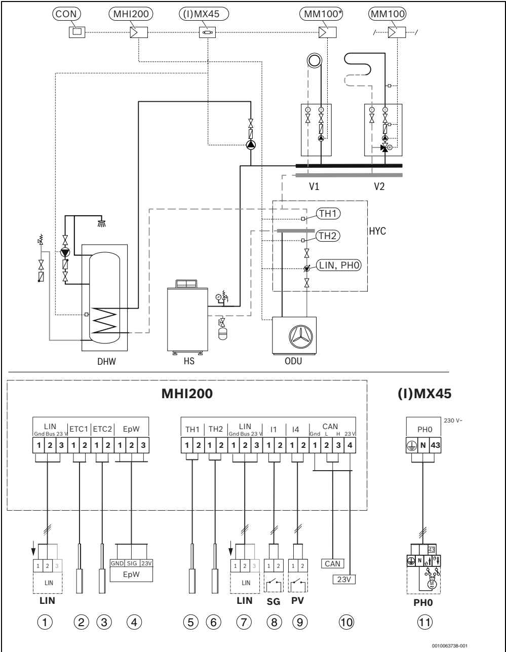
Afb. 25 Voorbeeld Hydraulisch systeem: Hybride systeem met vloerstaande cv-ketel, warm water aan ketel via laadpomp en 1-4 gemengde cv-circuits
