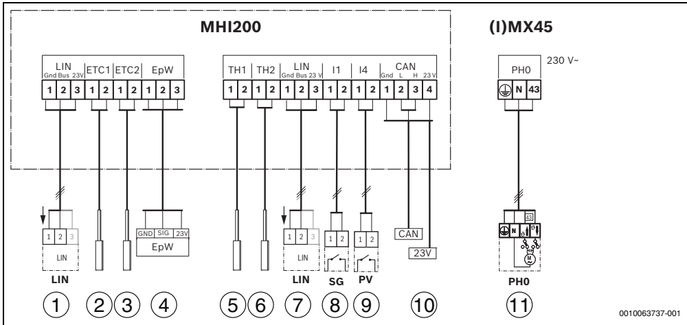
Bild 3 Überblick Anschlussklemmenbelegung
